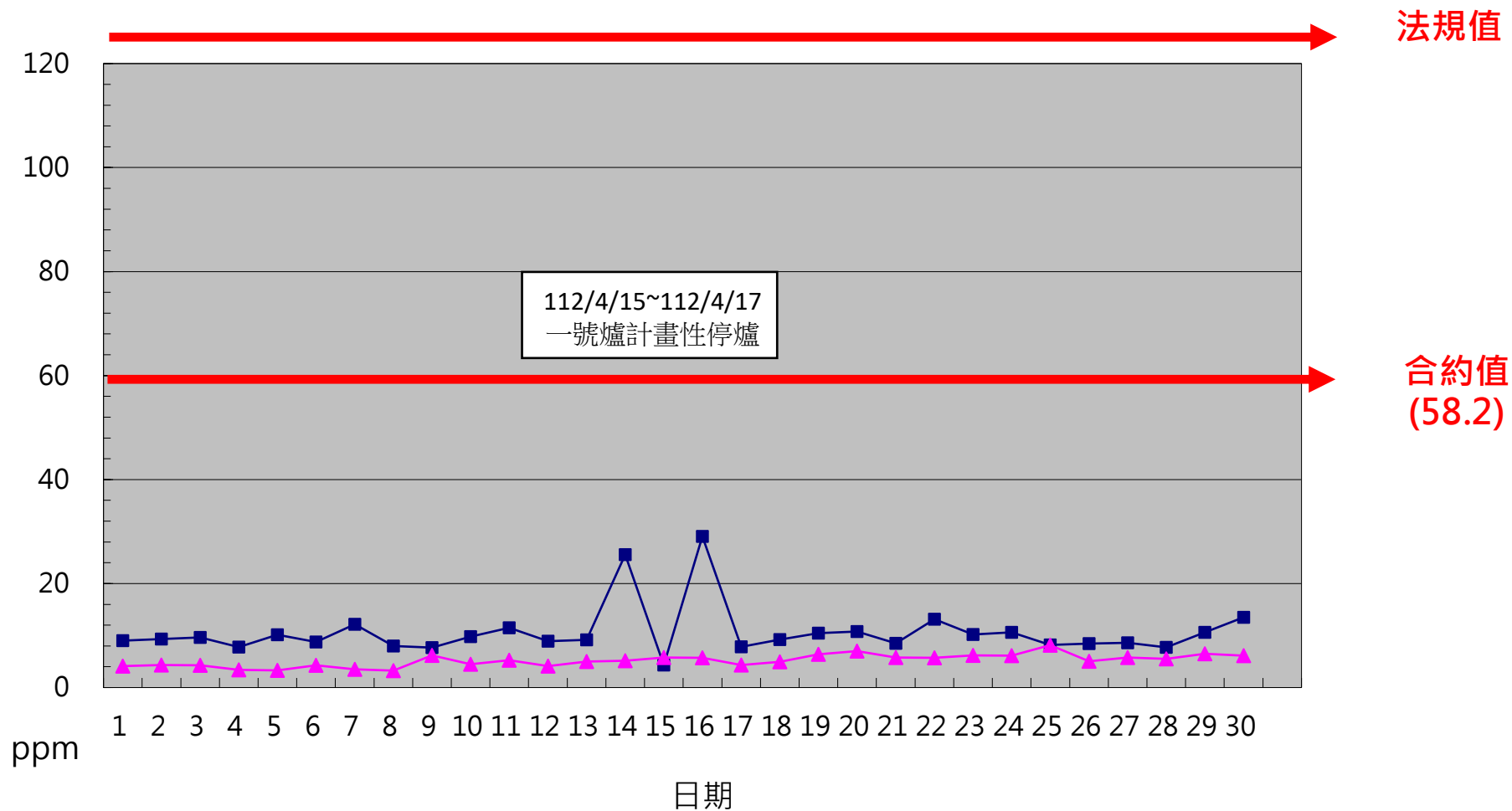
一百一十二年四月份 CO 單日24小時平均整月排放監測紀錄
