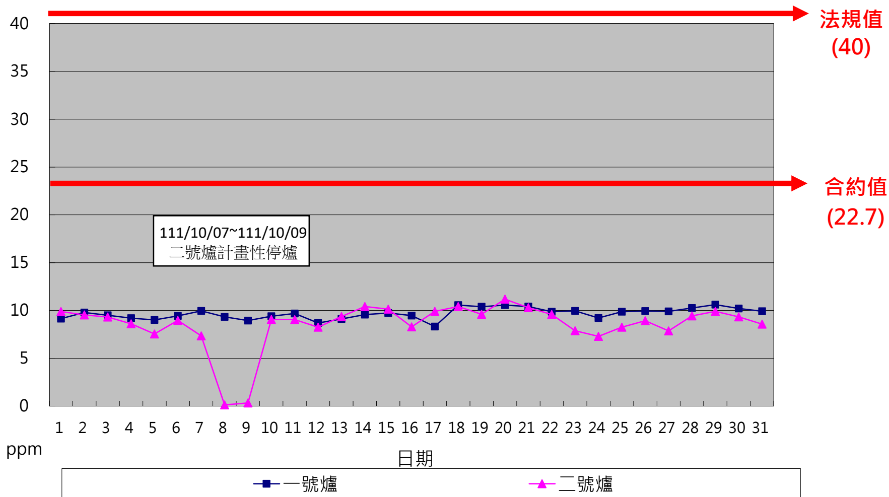
一百一十一年十月份 HCl單日24小時整月排放監測紀錄
