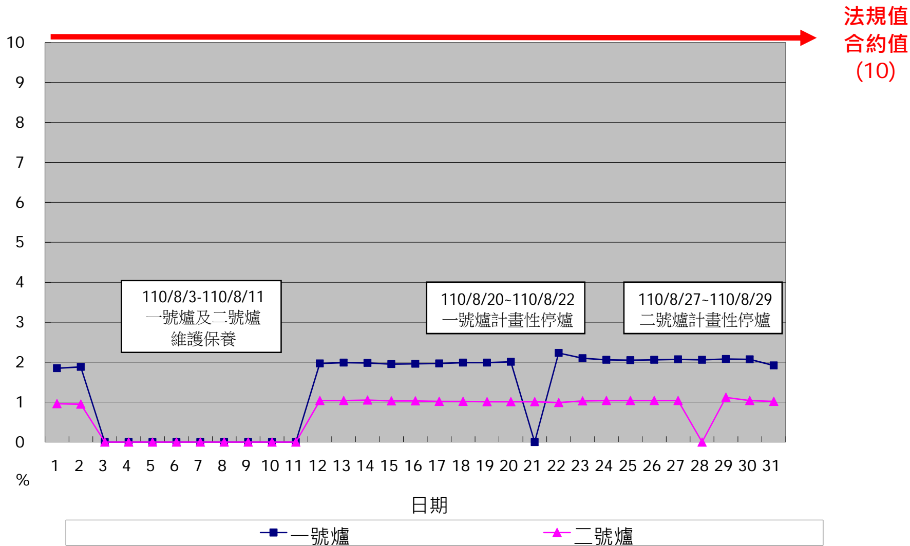
一百一十年八月份 OPACITY單日24小時整月排放監測紀錄
