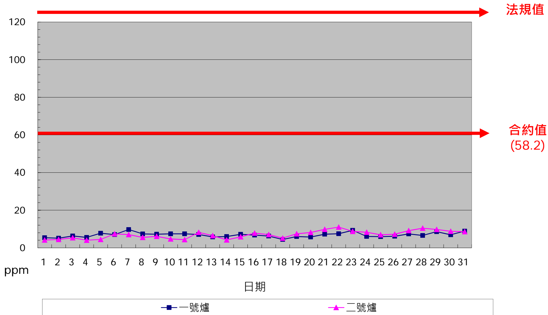
一百一十年七月份 CO單日24小時平均整月排放監測紀錄
