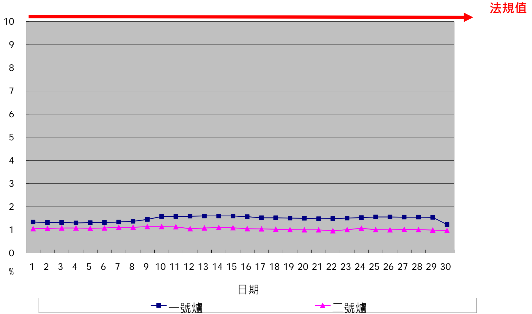
一百一十年六月份 OPACITY單日24小時整月排放監測紀錄
