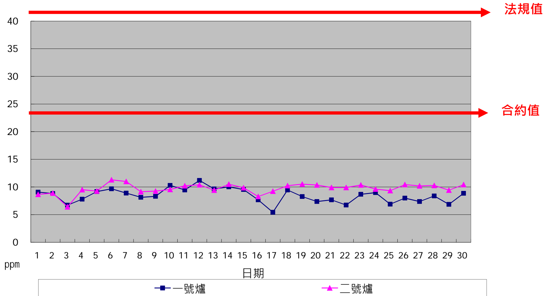
一百零九年六月份 HCl 單日24小時整月排放監測紀錄
