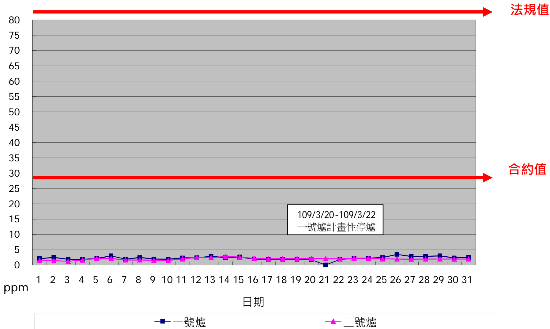
一百零九年三月份 SO x 單日24小時整月排放監測紀錄
