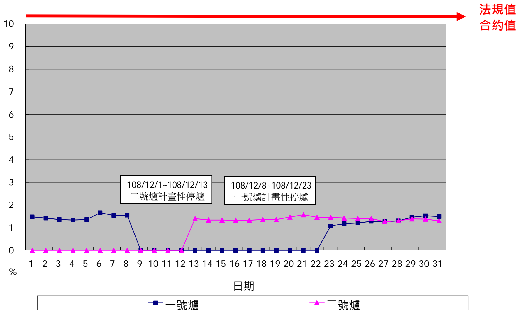
一百零八年十二月份 OPACITY 單日24小時整月排放監測紀錄
