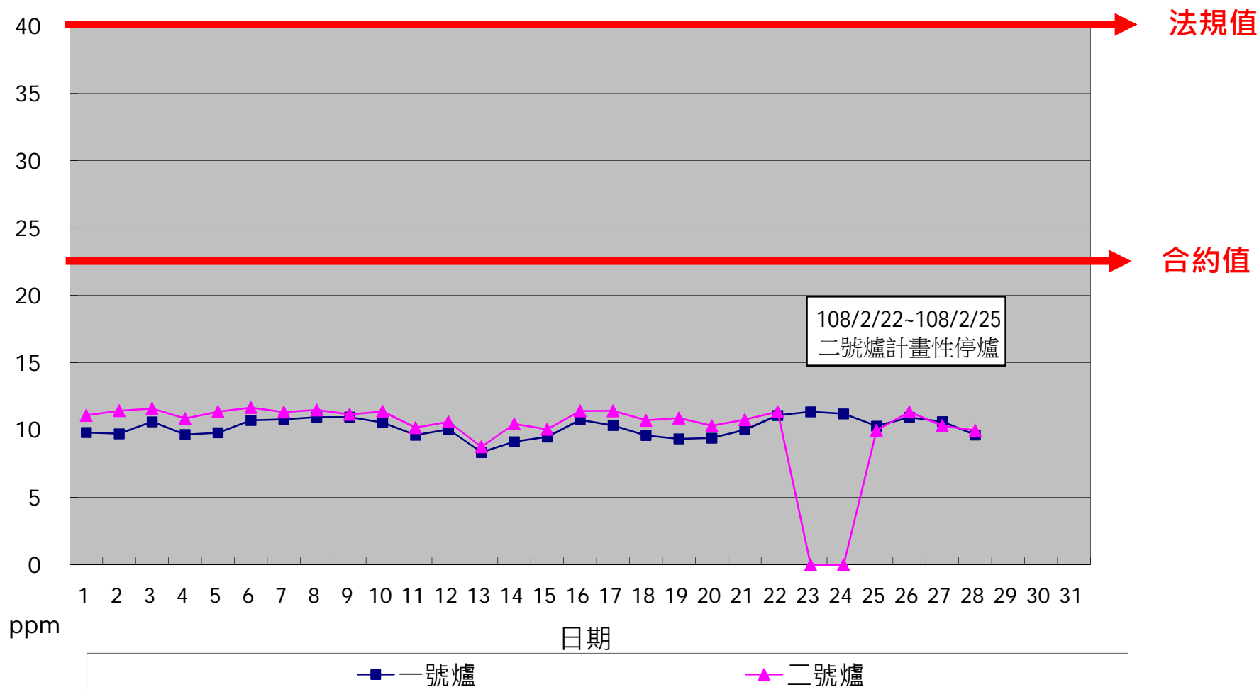
一百零八年二月份 HCl 單日24小時整月排放監測紀錄
