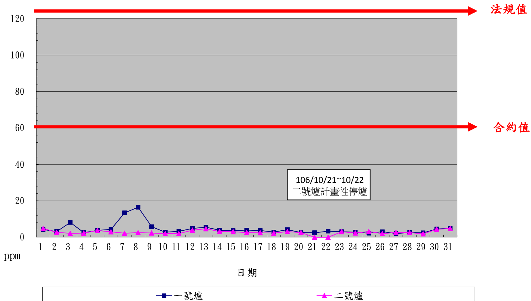
一百零六年十月份 CO 單日24小時平均整月排放監測紀錄
