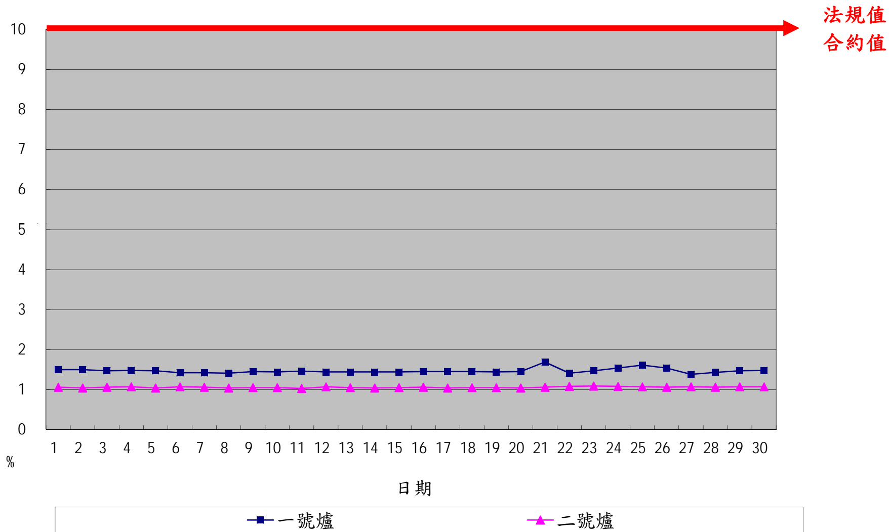
一百零五年六月份 OPACITY 單日24小時整月排放監測紀錄
