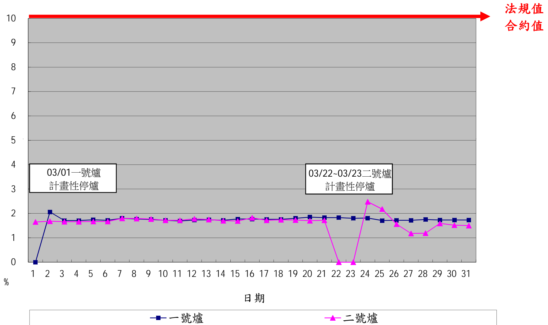
一百零三年三月份 OPACITY 單日24小時整月排放監測紀錄
